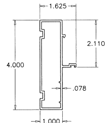
2 FRAME JAMB
